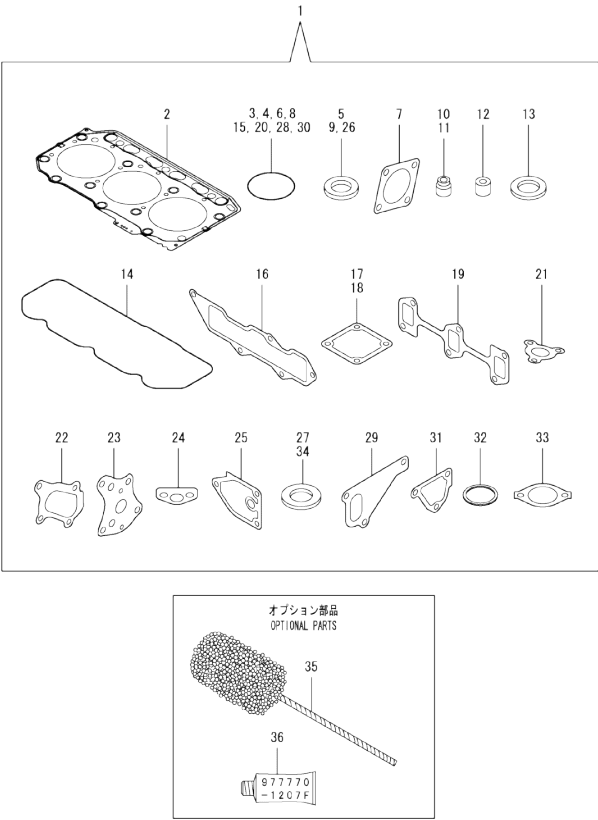
Fig.19. GASKET SET
